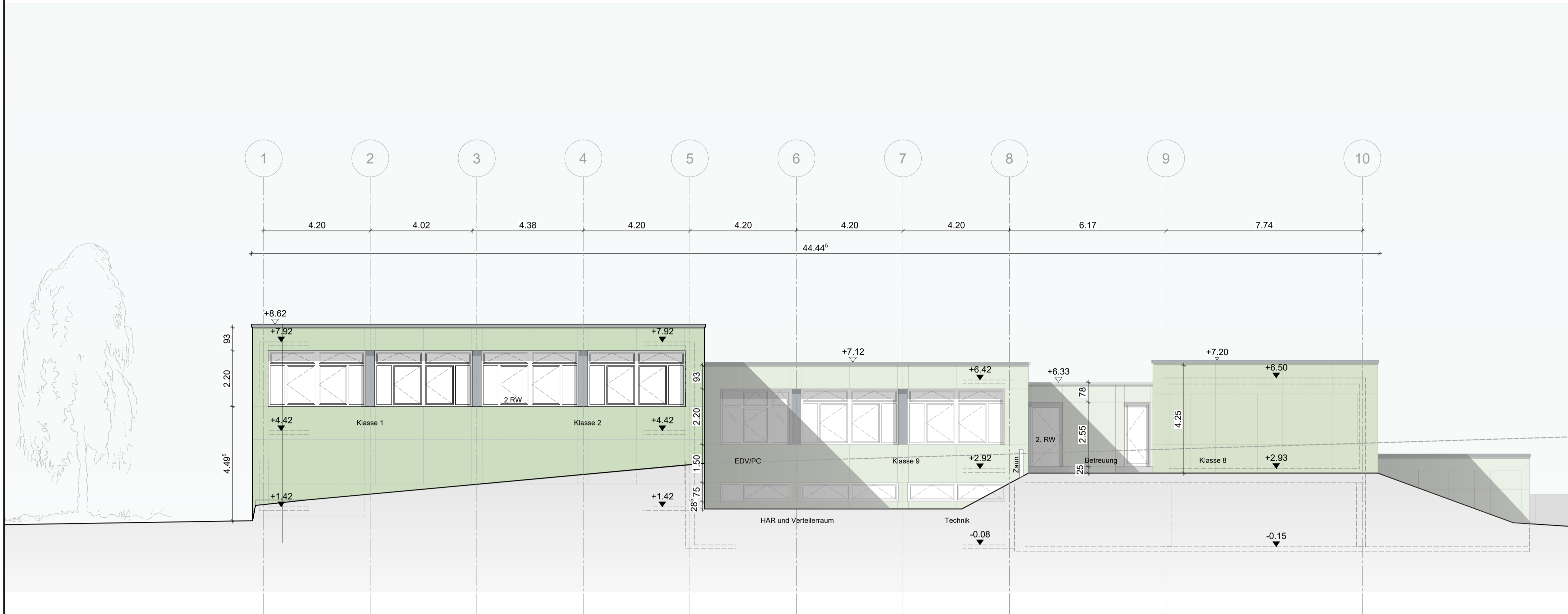
Ansicht Süd
